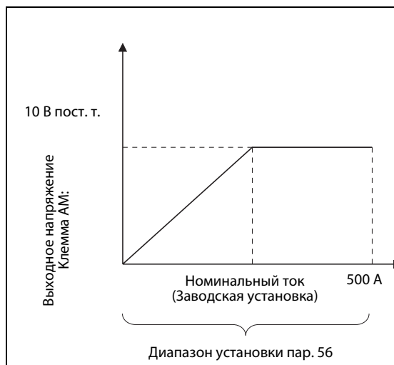
Рис. 6-74: Опорная величина для внешней индикации тока
