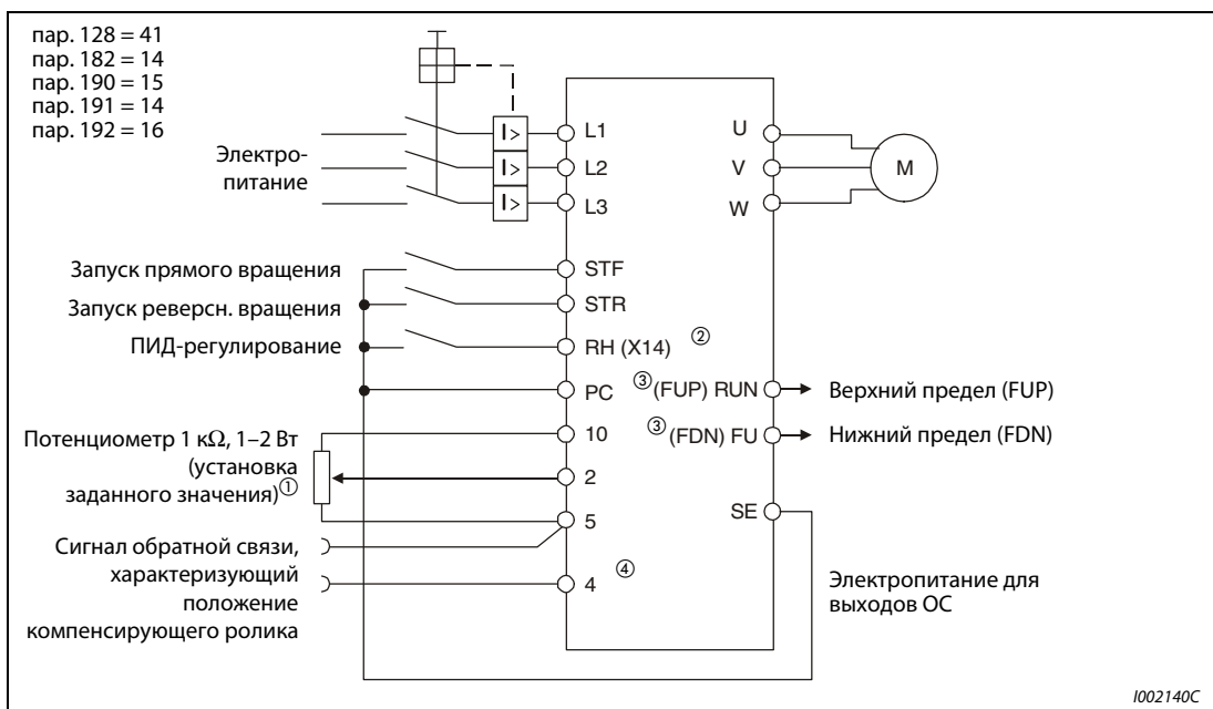
Рис. 6-146: Пример подключения при положительной логике
