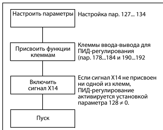
Рис. 6-141: Метод настройки
