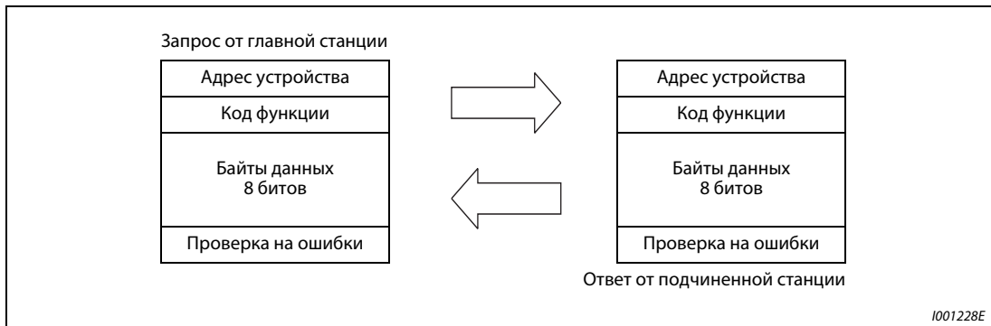
Рис. 6-130: Обмен данными
